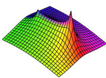
|\log \log(1-z)|
